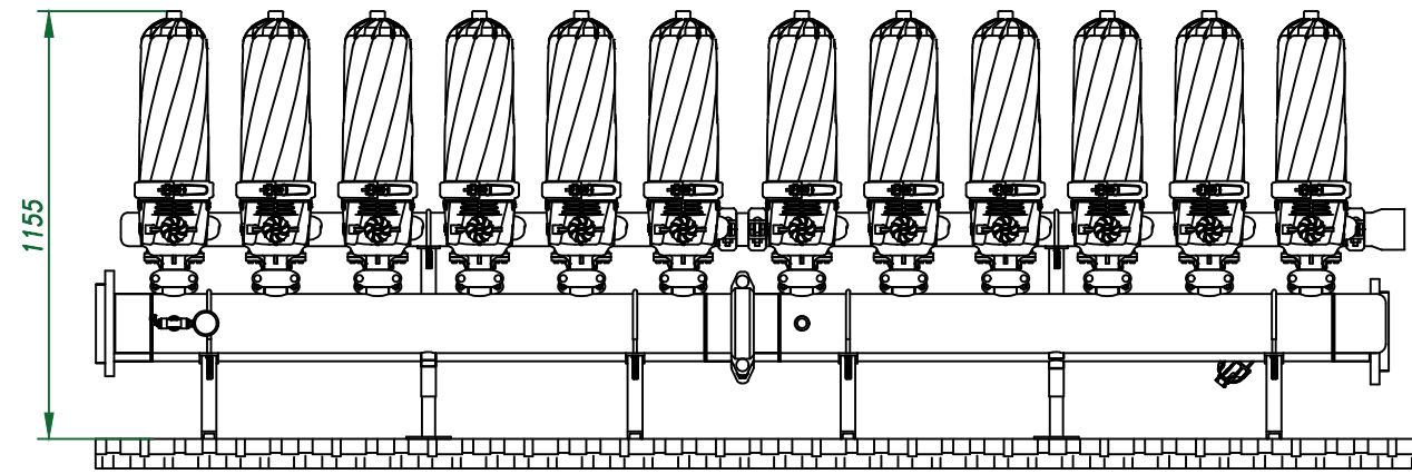
Вид спереди
